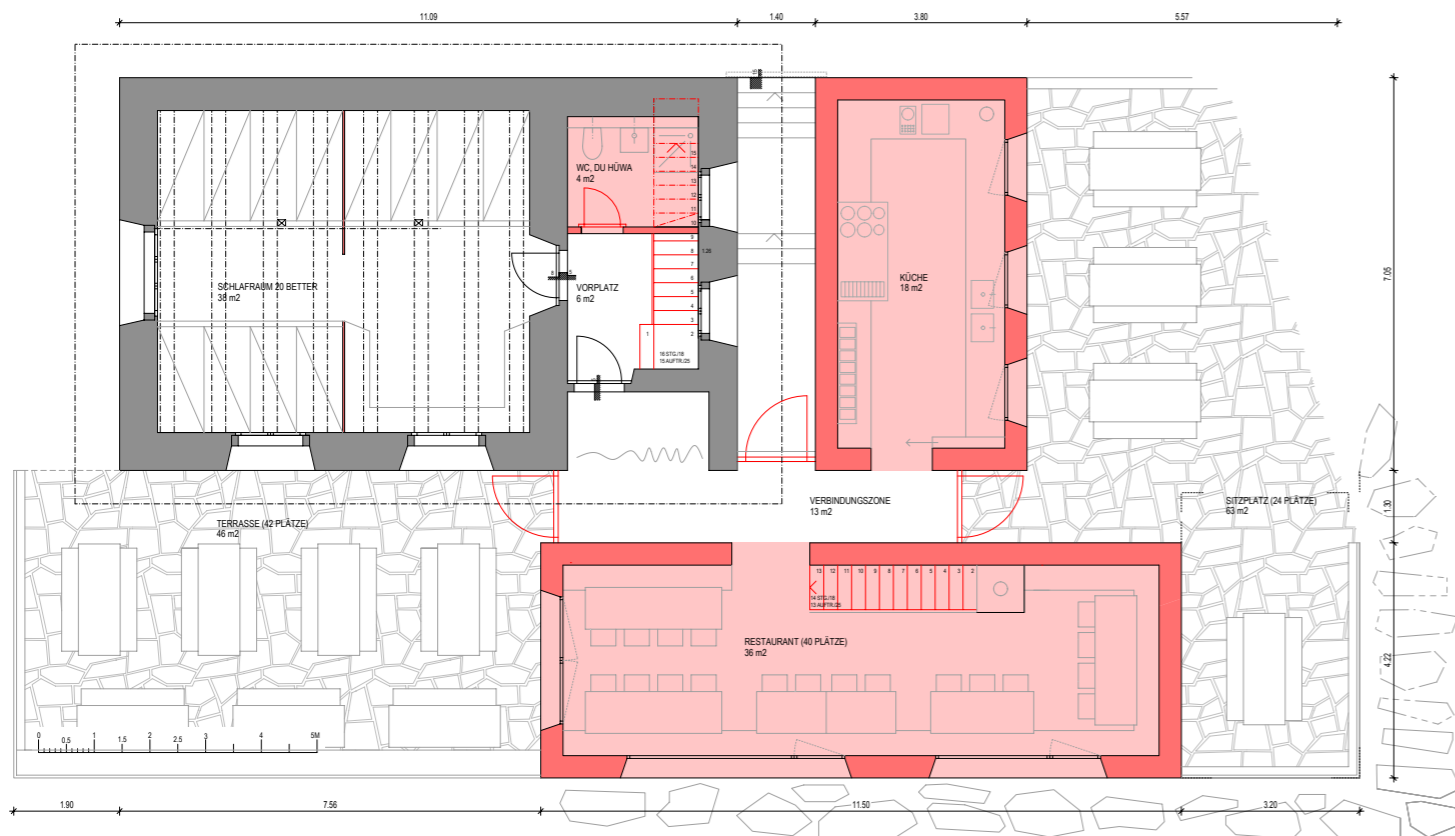
Grundriss Erdgeschoss
